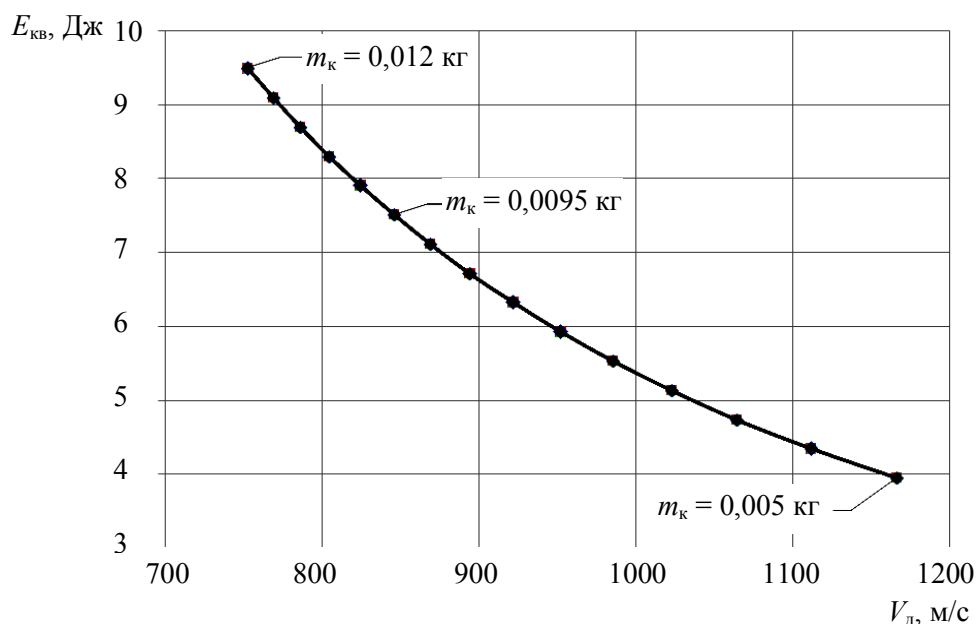
Рис. 2. Залежність енергії віддачі 7,62-мм СВД від дульної швидкості кулі при E_{кд} = 3400 Дж
