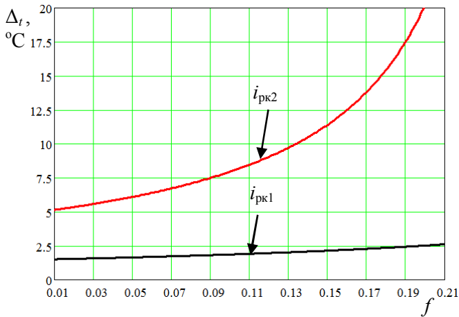
Рис. 5. Графік залежності \Delta_t = F(f, i_{рк}) \Big|_{f=0,02; \alpha=0}
