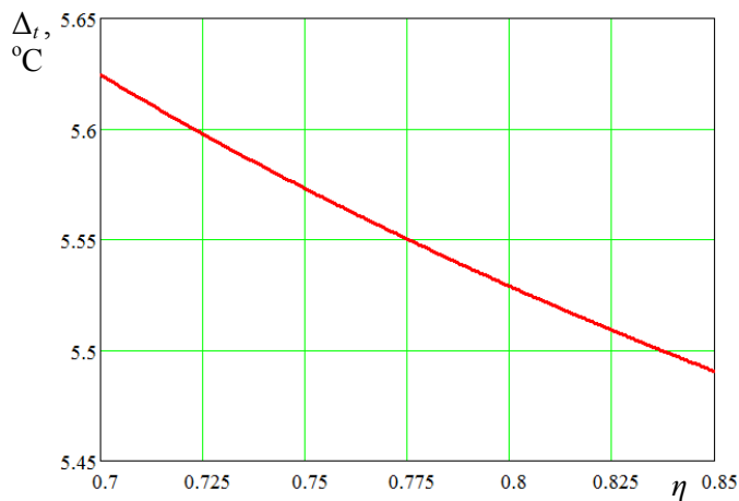
Рис. 4. Графік залежності \Delta_t = F(\eta_{тр}) \Big|_{f=0,02; \alpha=0}
