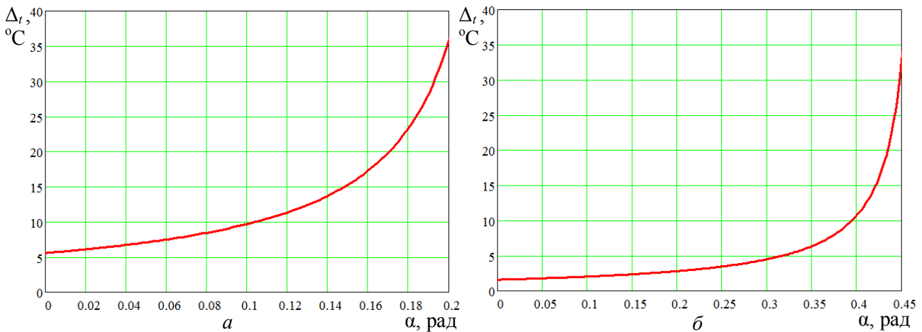
Рис. 6. Графік залежності \Delta_t = F(\alpha) \Big|_{f=0,02}
