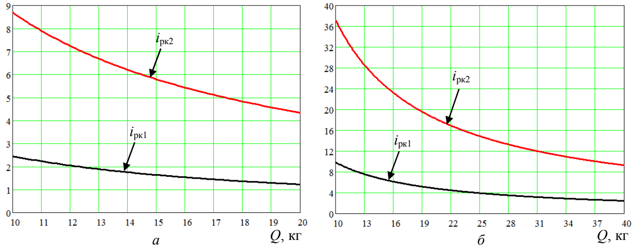
Рис. 3. Графік залежності \Delta_t = F(Q, i_{pk}) \Big|_{f=0,02; \alpha=0}
