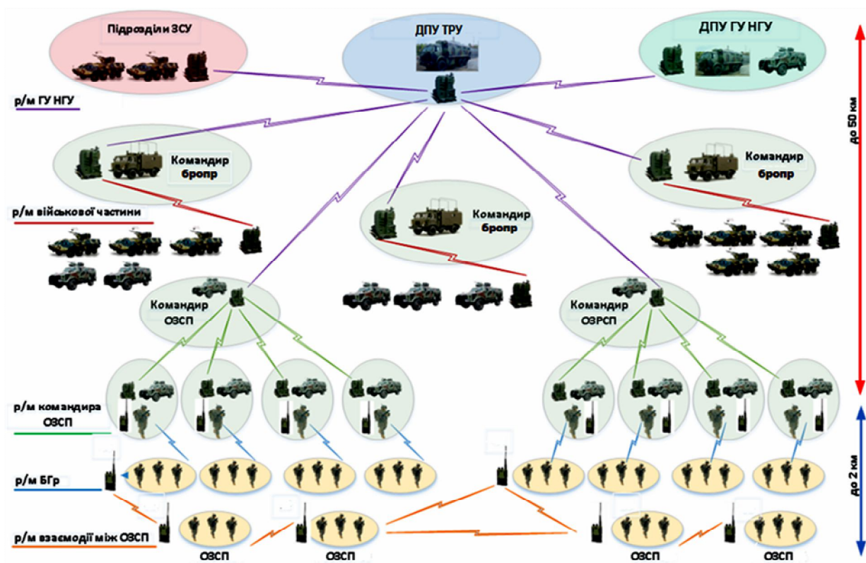
Рис. 1. Перспективна система радіозв'язку територіального управління Національної гвардії України (варіант)
