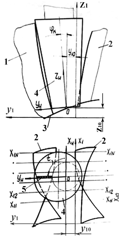
Рис. 1. До аналізу умов формоутворення каналової поверхні
