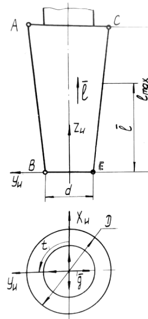
Рис. 3. Параметри кінцевої фрези з конічною ріжучою частиною
