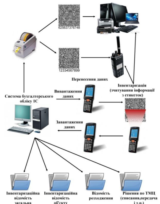
Рис. 3. Система інвентаризації за допомогою комп'ютерної техніки з використанням технології штрихового коду
