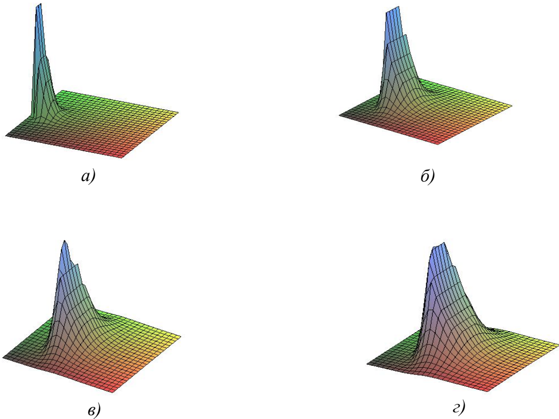
Рис. 1. Розподілення концентрації речовини для класу стійкості атмосфери А на різні моменти часу: а) t = 1 с; б) t = 3 с; в) t = 5 с; г) t = 10 с
