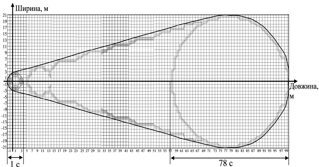
Рис. 2. Результати моделювання зони ураження
